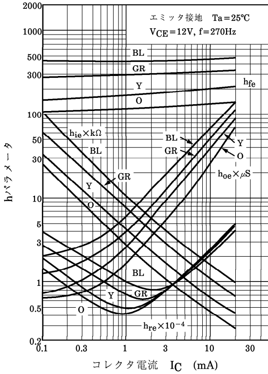
hパラメータ - I_C
