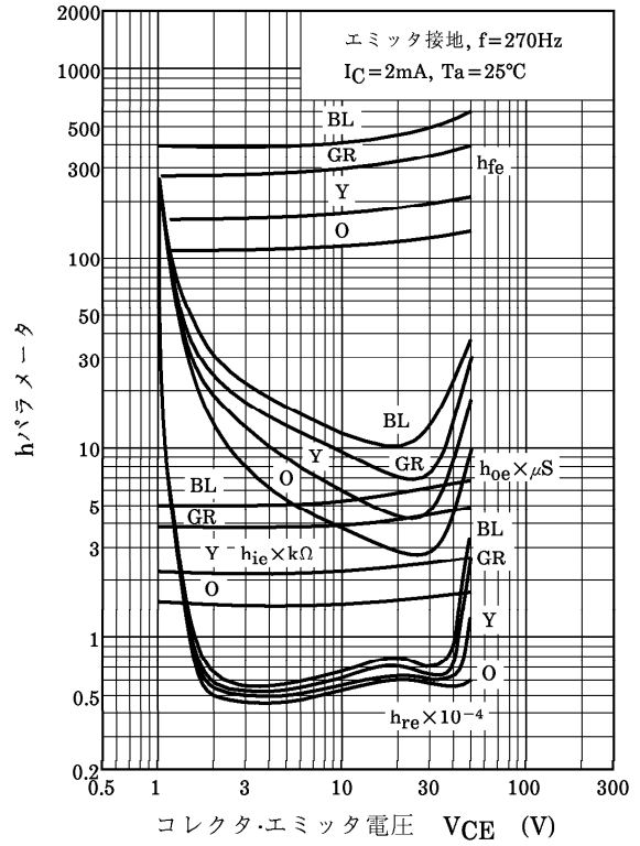
hパラメータ - V_{CE}
